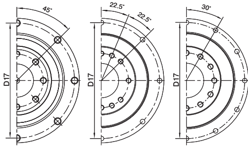
图示为带平键的 PSFNpro090 / 1 级 / 法兰输出轴 / 14 mm 锁紧系统 / 适配电机法兰 - 2 件式 - 圆形通用法兰 / B5 电机法兰类型 Drawing corresponds to a PSFNpro090 / 1-stage / flange output shaft / 14 mm clamping system / motor adaptation - 2-part - round universal flange / B5 flange type motor
