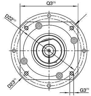
图示为带平键的 PSFNpro090 / 1 级 / 法兰输出轴 / 14 mm 锁紧系统 / 适配电机法兰 - 2 件式 - 圆形通用法兰 / B5 电机法兰类型 Drawing corresponds to a PSFNpro090 / 1-stage / flange output shaft / 14 mm clamping system / motor adaptation - 2-part - round universal flange / B5 flange type motor
